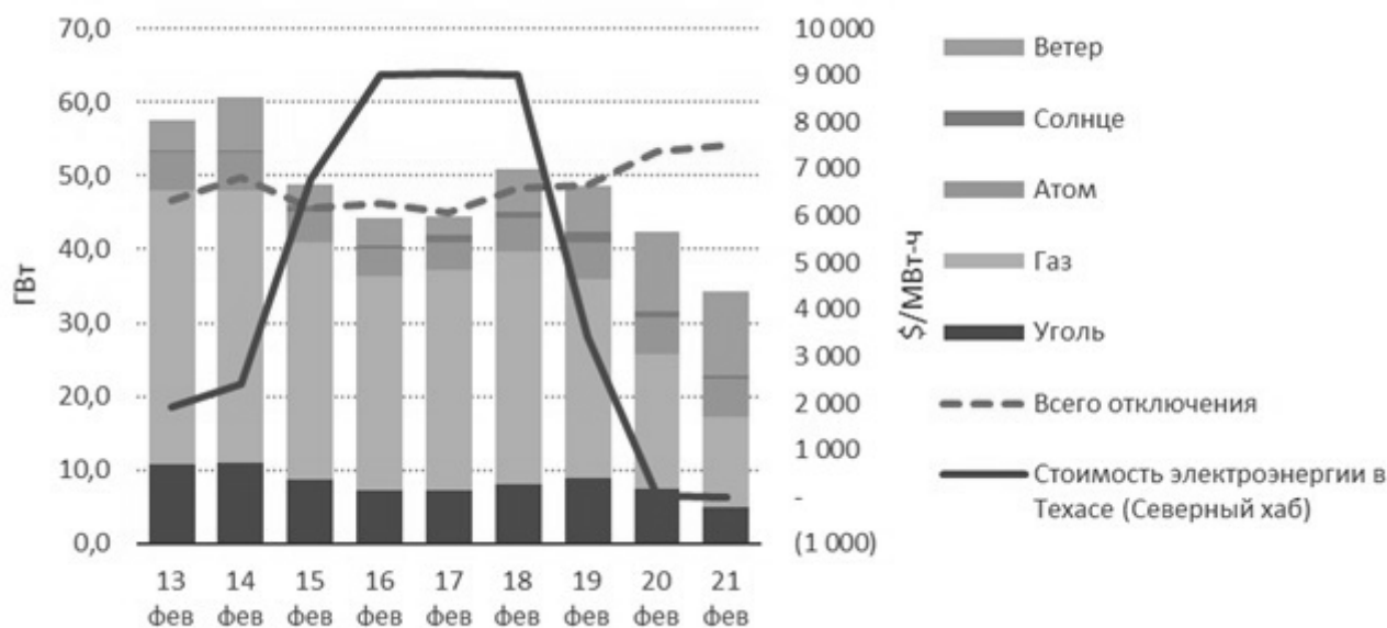
Рис. 8 / Fig. 8. Влияние веерных отключений и динамики электрогенерации по типу топлива в штате Техас на стоимость электроэнергии в реальном времени в период холодов (фев. 21 г.) / Impact of rolling blackouts and power generation dynamics by fuel type in Texas on real-time electricity costs during cold weather (Feb 21)
