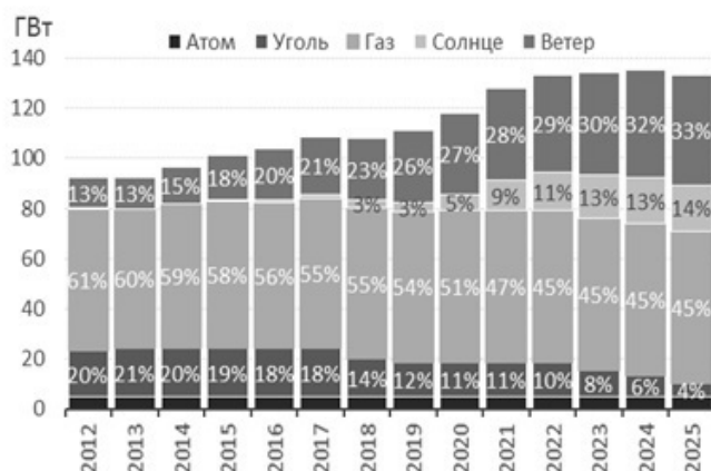
Рис. 5 / Fig. 5. Изменение структуры электрогенерации* в Штате Техас по типу топлива 2012–2020 гг. и прогноз на 2021–2025 гг. / Change in the structure of electricity generation* in the State of Texas by type of fuel 2012–2020 and forecast for 2021–2025
